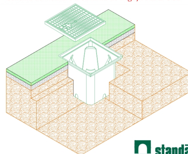
Schema de montare a căminul de irigații PIPE CUB
