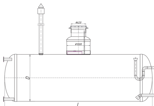
Gama dimensională a Rezervoarelor TankLine TLD subterane pentru apă potabilă Габаритные размеры резервуаров питьевой воды TankLine TLD
